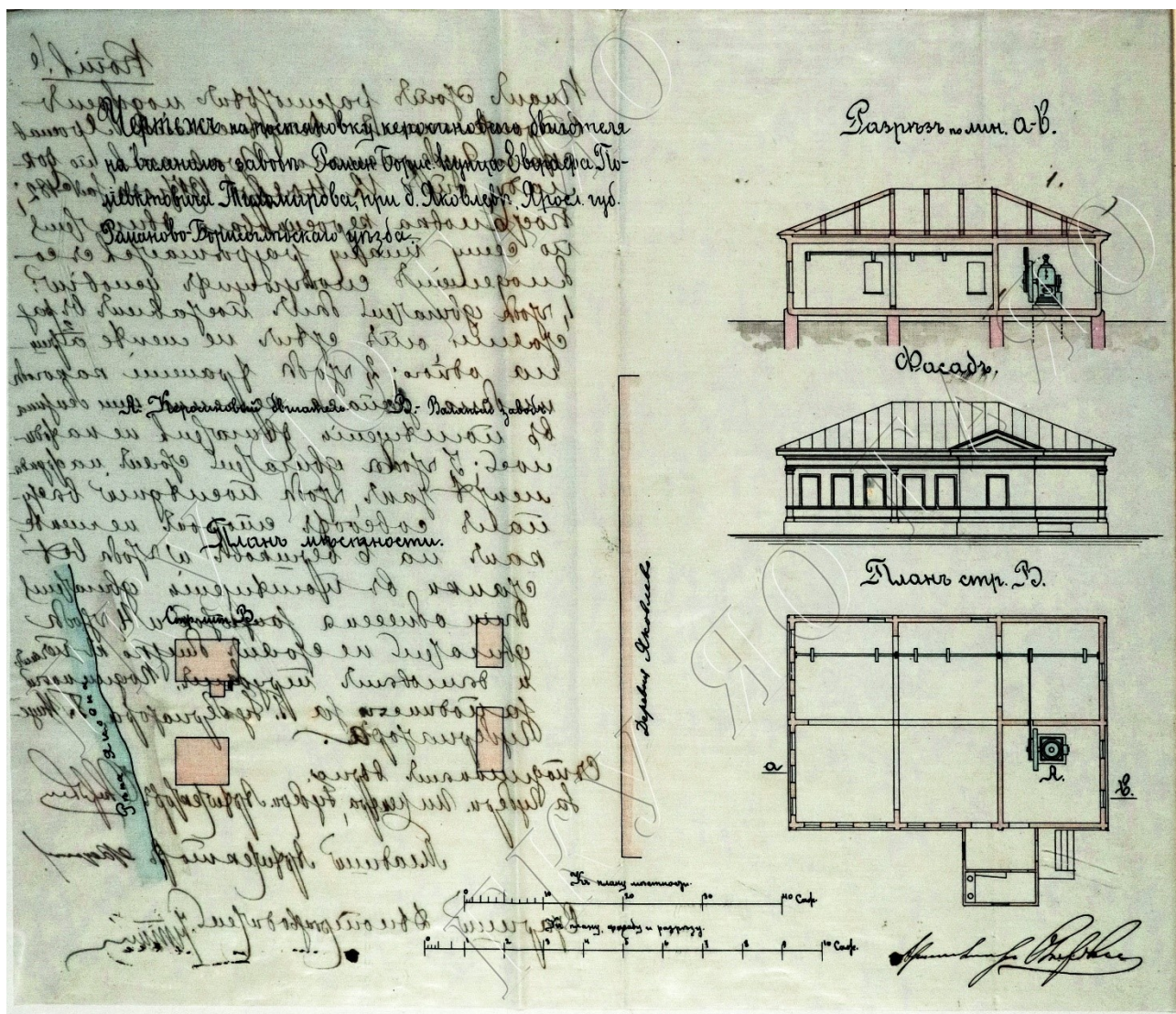
Чертеж на постановку керосинового двигателя на валяном заводе купца Е.П. Тихомирова при деревне Яковлево Романово-Борисоглебского уезда Ярославской губернии. 1897 г. ГКУ ЯО ГАЯО. Ф. 80. Оп. 1. Д. 1245. Л. 6 об.
